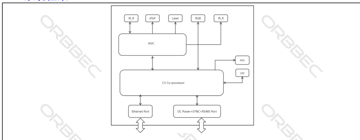
图 4-3-1 Gemini 435Le 相机系统框图
